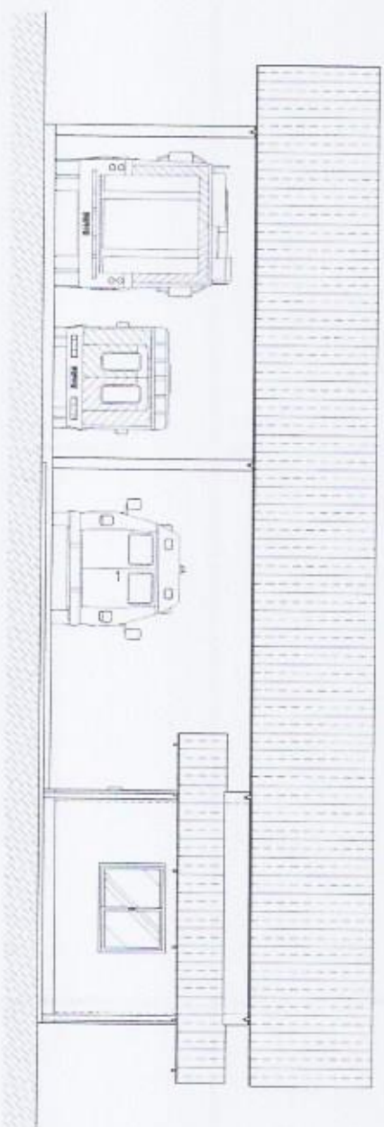
แบบรูปด้าน 3
